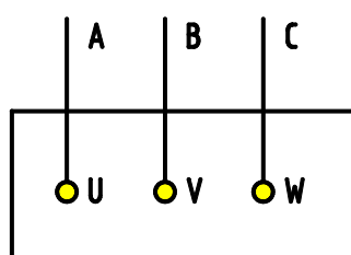
风机接线
